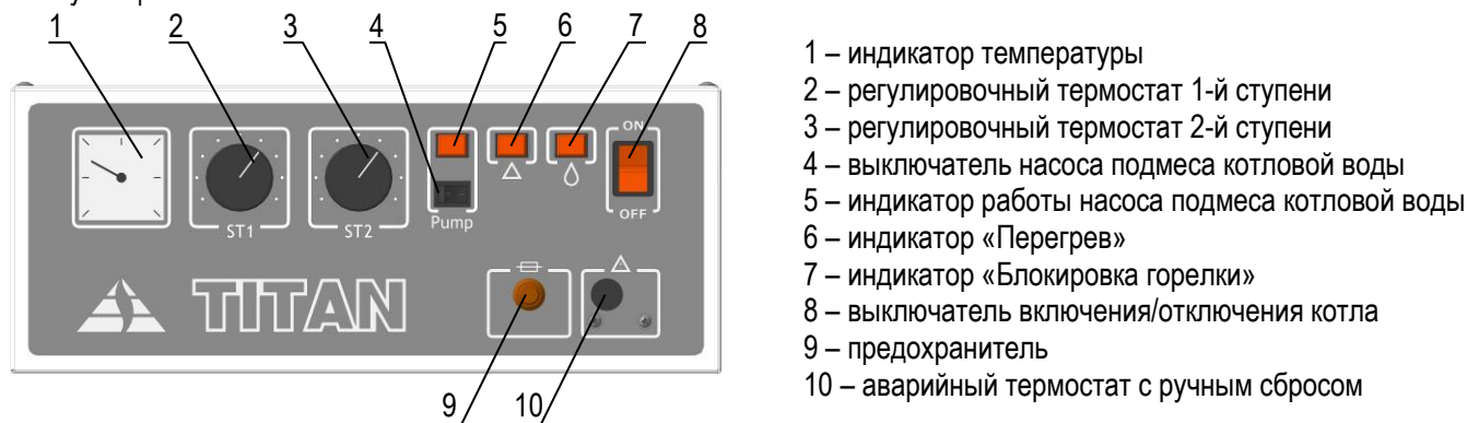
Рисунок 6. Внешний вид панели управления котла
