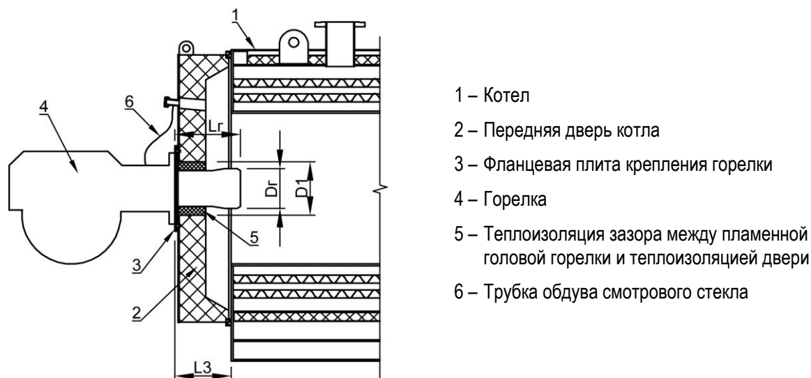
Рисунок 4. Установка горелки
